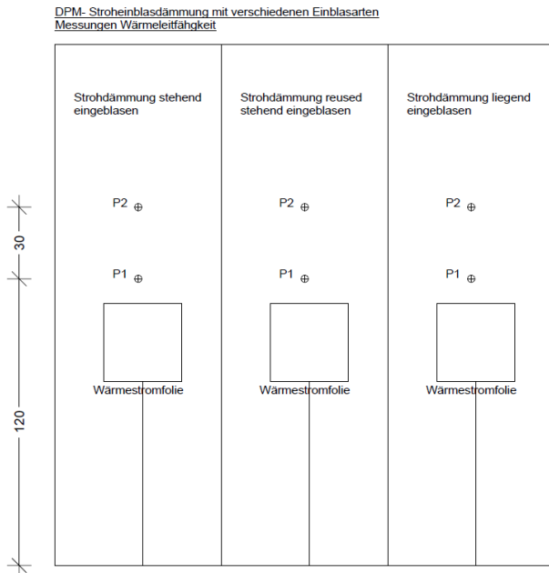
Abbildung 1: Messpunkte Positionen
